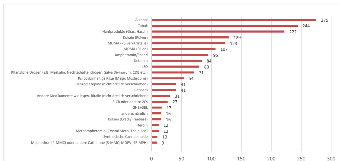
Abb.1: 12-Monats-Prävalenz, n=298
